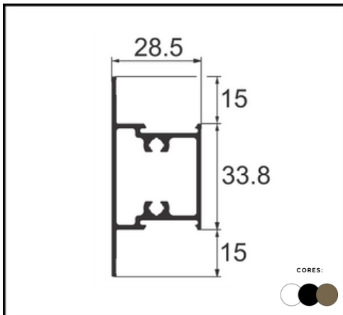
PERFIL LG 055 TRAVESSA GOLD
