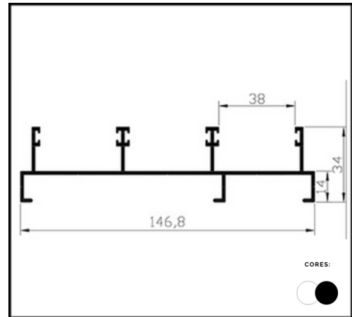
PERFIL LG 064 LATERAL 3 PLANOS GOLD
