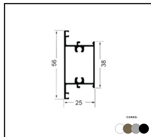
PERFIL P 319 TRAVESSA
