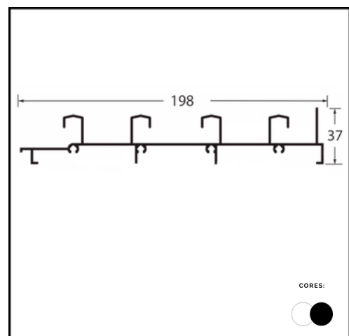
PERFIL LG 071 TRILHO 4 VIAS GOLD
