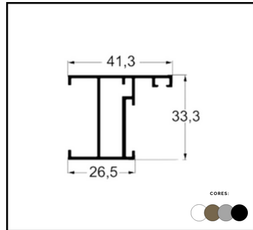
PERFIL SU 279 CONTRA MARCO
