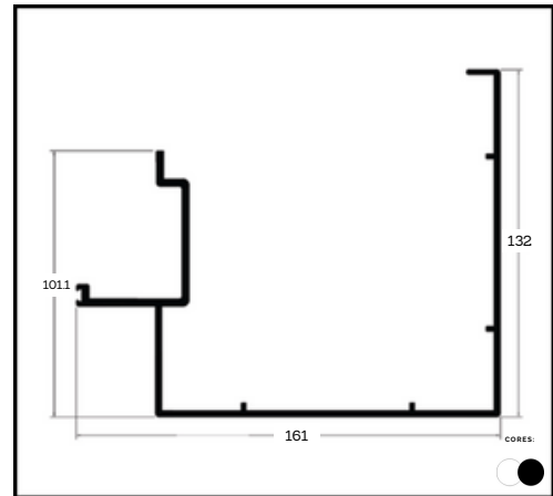
PERFIL EPO 113 CAIXA DO PORTAO
