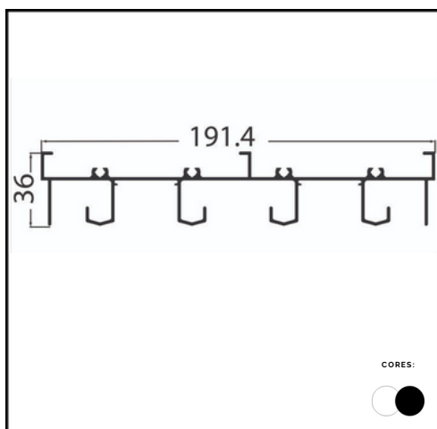
PERFIL LG 070 TRILHO 4 VIAS GOLD
