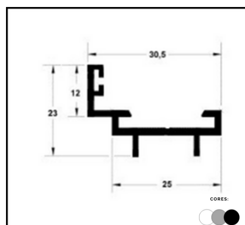
PERFIL L 715 CONTRA MARCO
