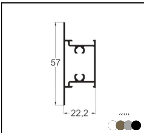
PERFIL SU 227 TRAVESSA
