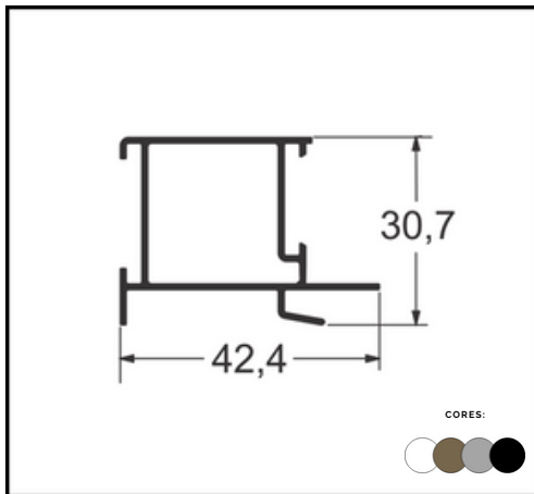
PERFIL SU-047 BITUBULAR
