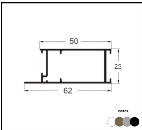
PERFIL SU 111 MONTANTE
