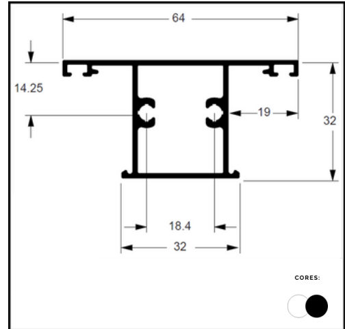
PERFIL LG 083 MARCO FOLHA FIXA GOLD
