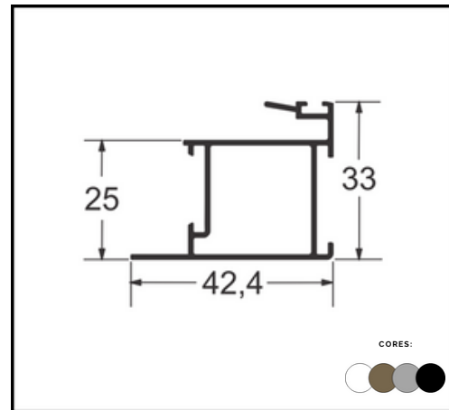
PERFIL SU-049 BITUBULAR
