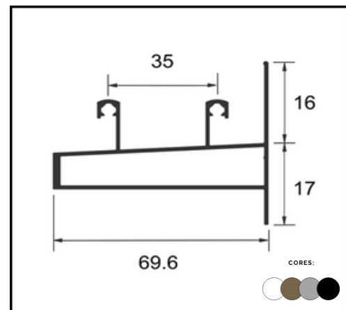
PERFIL SU-006 TRAVESSA DE BANDEIRA
