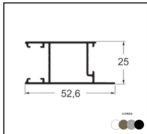
PERFIL SU-039 MONTANTE VERTICAL
