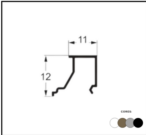
PERFIL SU- 102 BAGUETE CURTA JANELA
