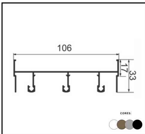
PERFIL SU 010 TRILHO TRIPLO
