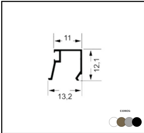
PERFIL P 414 FOLHA PORTA
