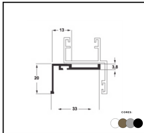
PERFIL L 387 PINGADEIRA
