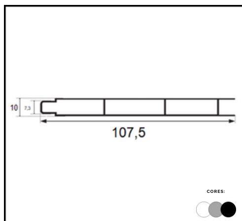
PERFIL LB 600 LAMBRI DUPLO
