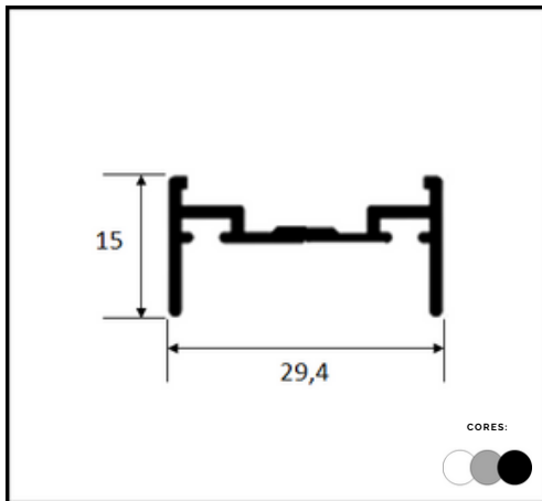
PERFIL P 140 FOLHA DE JANELA
