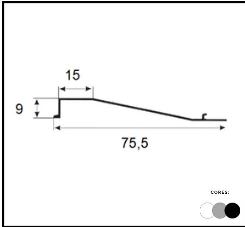
PERFIL US 280 VENEZIANA VAZADA
