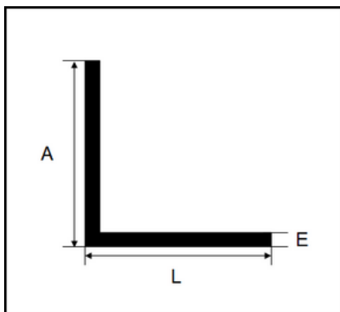
PERFIL CT CANTONEIRA ESTRUTURAL "L"
