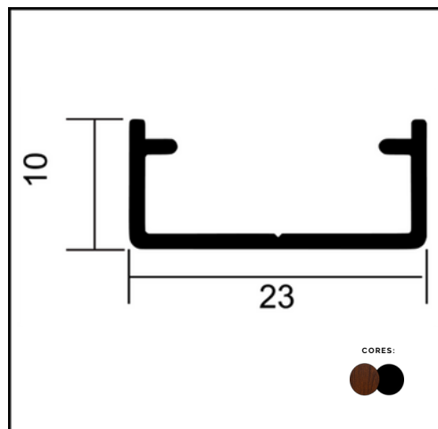
PERFIL MUXARABI 31-128 C - PERFIL U
