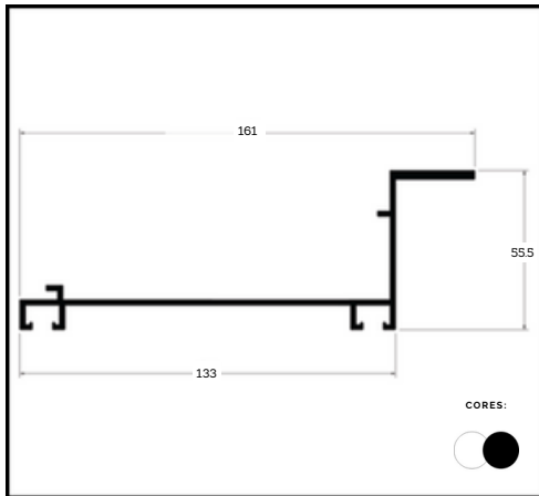
PERFIL EPO 112 TAMPA DA CAIXA DO PORTAO
