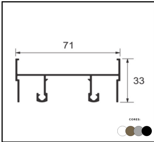
PERFIL SU-003 MARCO LATERAL
