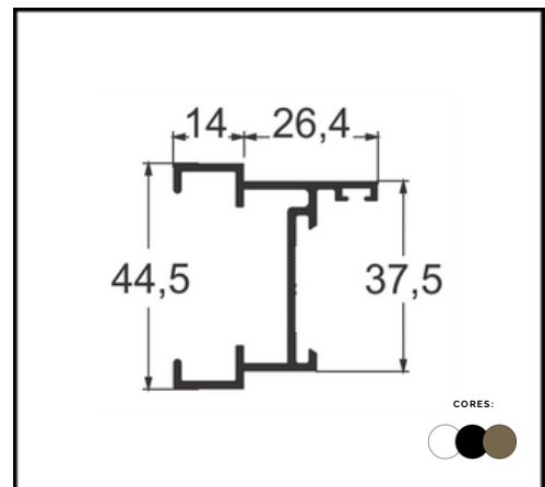
PERFIL LG 059 BAGUETE LARGO GOLD
