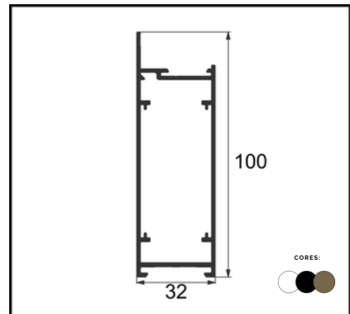
PERFIL LG 042 MOLDURA DA PORTA GOLD
