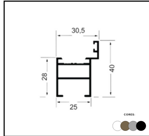
PERFIL P 153 TRAVESSA MENOR
