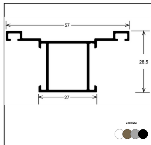
PERFIL SU-085 TRAVESSA/MARCO
