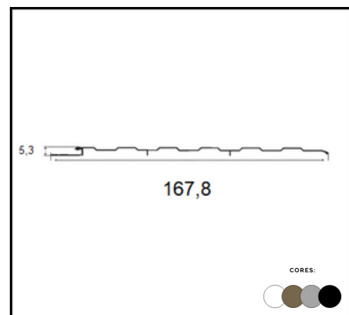
PERFIL LB 050 LAMBRI FRISADO
