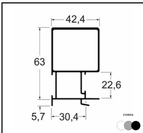
PERFIL SU- 053 TRAVESSA INF/SUP
