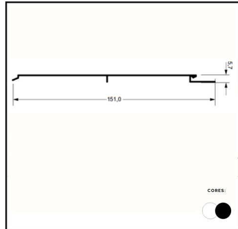
PERFIL LB 088 LAMBRI LISO LISO
