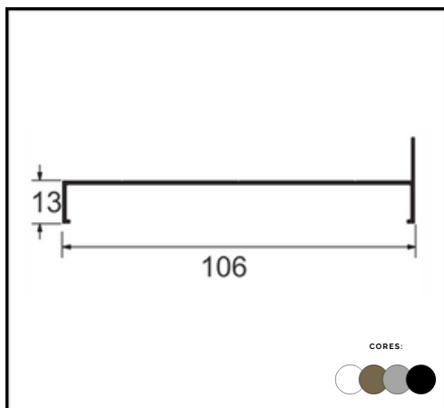
PERFIL SU 012 CONTRA MARCO
