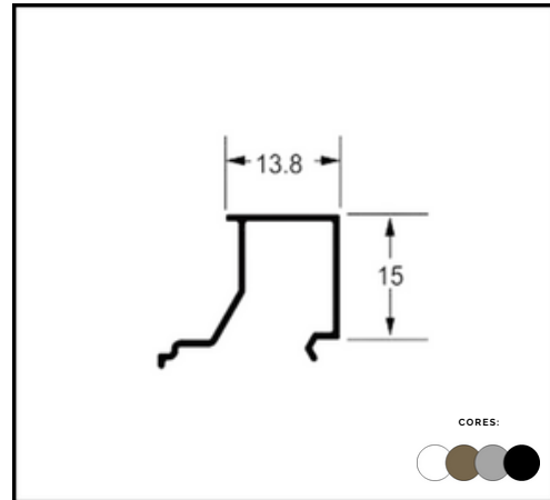
PERFIL SU- 103 BAGUETE LARGA
