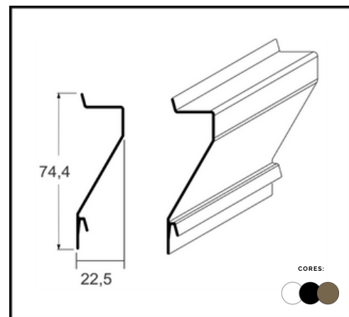
PERFIL VZ 047 - VENEZIANA (COM OLHAL)
