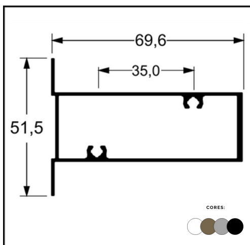
PERFIL SU-009 - COLUNA
