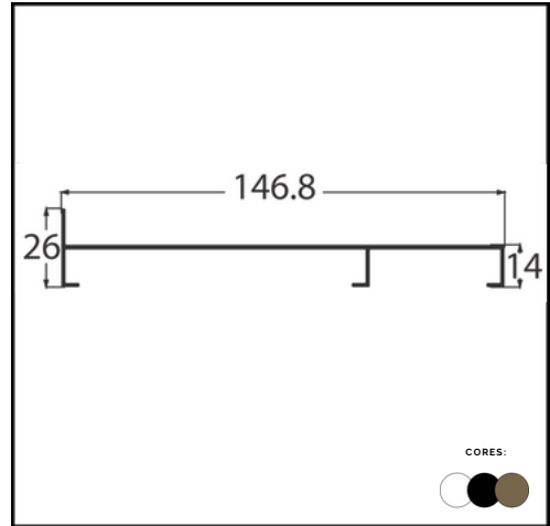
PERFIL LG 158 - LATERAL 3 PLANOS GOLD
