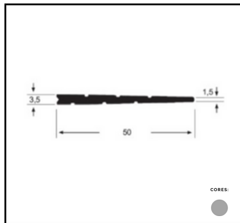
PERFIL S 0116 - CUNHA NATURAL 03 METROS
