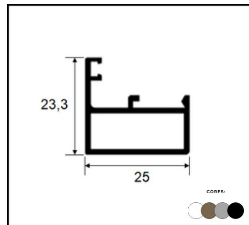
PERFIL P 147 BANDEIRA
