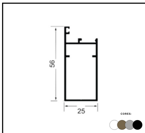
PERFIL P 318 FOLHA PORTA
