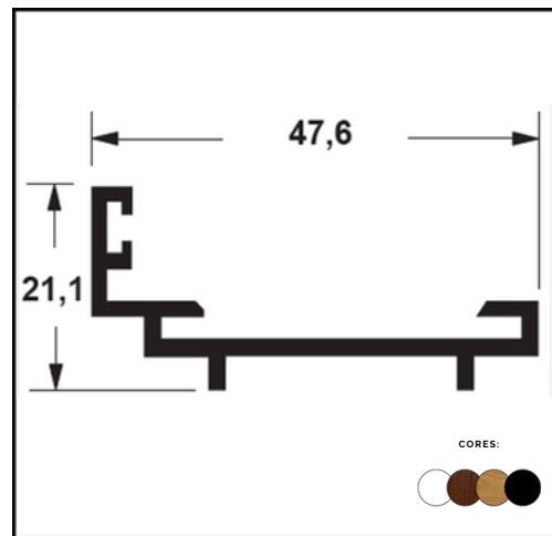
PERFIL L-521
