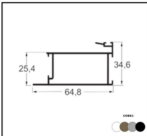
PERFIL SU 242 MÃO AMIGA PORTA
