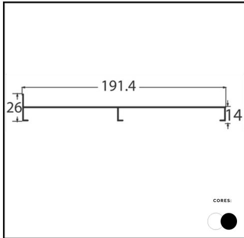
PERFIL LG 077 INVERSO BAGUETE GOLD
