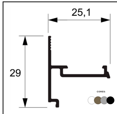
PERFIL SU- 292 - REVERSOR DE BAGUETE
