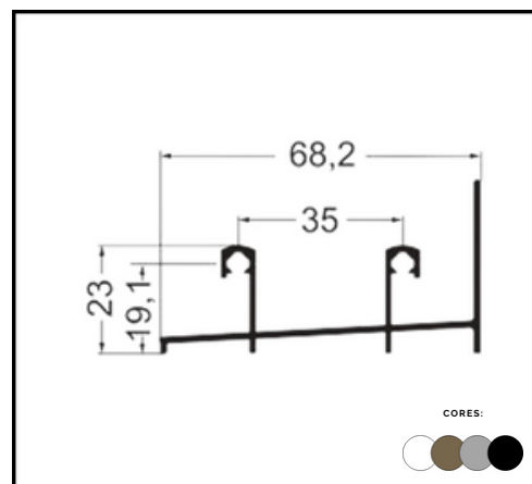
PERFIL SU 228 TRILHO PORTA
