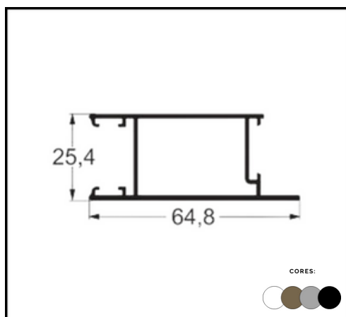
PERFIL SU 245 PORTA DE CORRER
