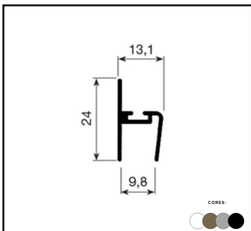
PERFIL AL 17 CADEIRINHA
