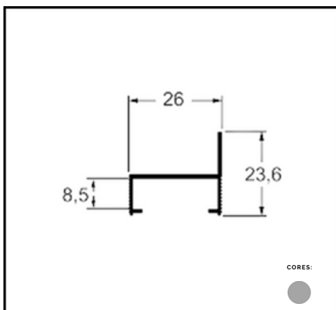
PERFIL CM 200 ARREIMATE
