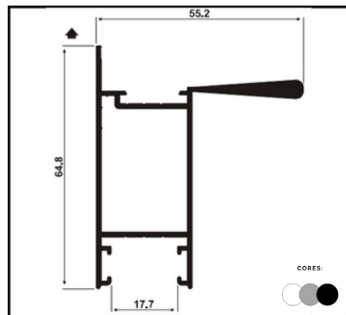
PERFIL SU-085 TRAVESSA/MARCO
